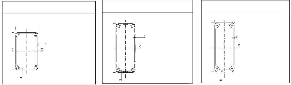
Sezione arcata tipo e di testata
